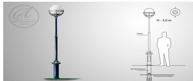
T/X по теме: Фонарь ЛУНЬ Н - 3,0 м. Материал: Опора: Сталь - (С15ГС, 08ГС). Рассеиватель: Шар 400 (Полим Сталь - (С15ГС, 08ГС)). Грунт: - Эмаль 3в1 (антикоррозийный). Краска: Forgent Paint (Синий). Патина: WS - Patina (под Золото). Электрокомплектация: E 27. ПВС 3X1,5. BA47 -29. ЗНИ-16. Для индивидуального подхода по теме Т/Х контакт с производством тел. факс: (8652) 23 04 81. (8652) 22 04 41.
