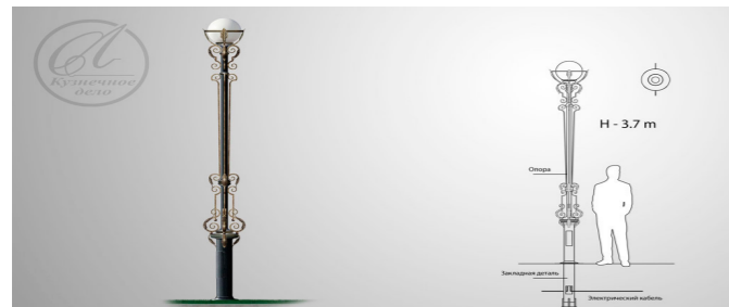
T/X по теме: Фонарь Велес. Н - 3,7 м. Материал: Опора: Сталь - (С15ГС, 08ГС). Рассеиватель: Шар 400 (Полим Сталь - (С15ГС, 08ГС)). Грунт: - Эмаль 3в1 (антикоррозийный). Краска: Forgent Paint (Черный). Патина: WS - Patina (под Золото). Электрокомплектация: E 27. ПВС 3X1,5. BA47 -29. ЗНИ-16. Для индивидуального подхода по теме Т/Х контакт с производством тел. факс: (8652) 23 04 81. (8652) 22 04 41.
